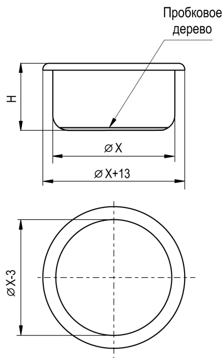
Подстаканник ИАРС. 301171.002
